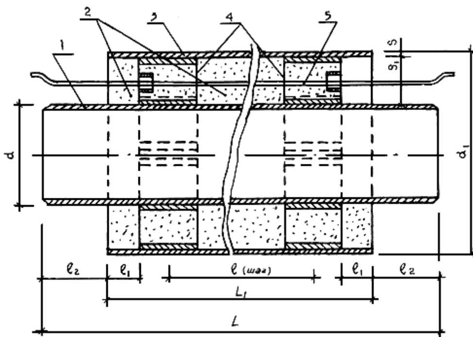
Рис. 1. Индустриальная конструкция теплоизоляции:
